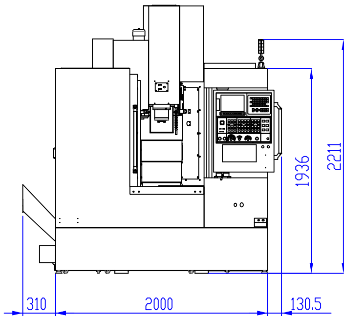
V-30IF 外型尺寸圖
